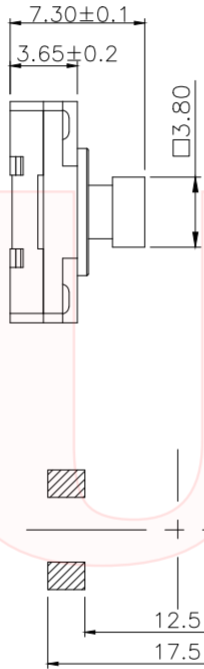
PCB Layout(Pattern side)
